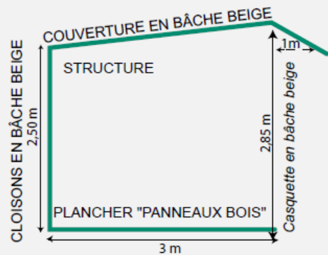
Module toilé couvert 9 m 2 (3x3)
