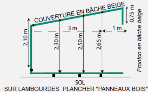
Module toilé couvert 9 m 2 (3x3)
